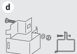
počiatočná objímka
